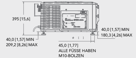
Seitenansicht
